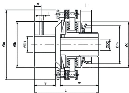
Rutschkupplung ECSK für direkte Antriebe
