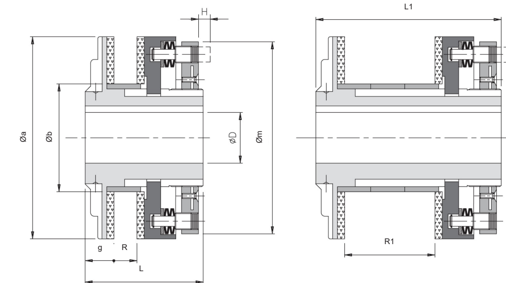
Rutschkupplung ECS für indirekte Antriebe ab Größe 4800 links mit kurzer Nabe / rechts mit langer Nabe
