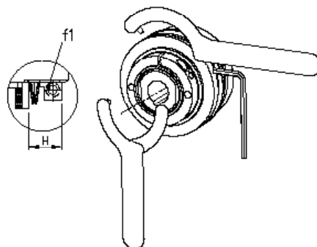
Nabe mit radialer Sicherung
